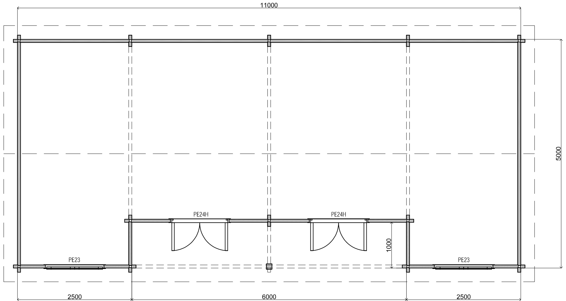
Plattegrond / Plan
