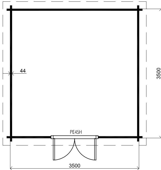
Plattegrond / Plan
